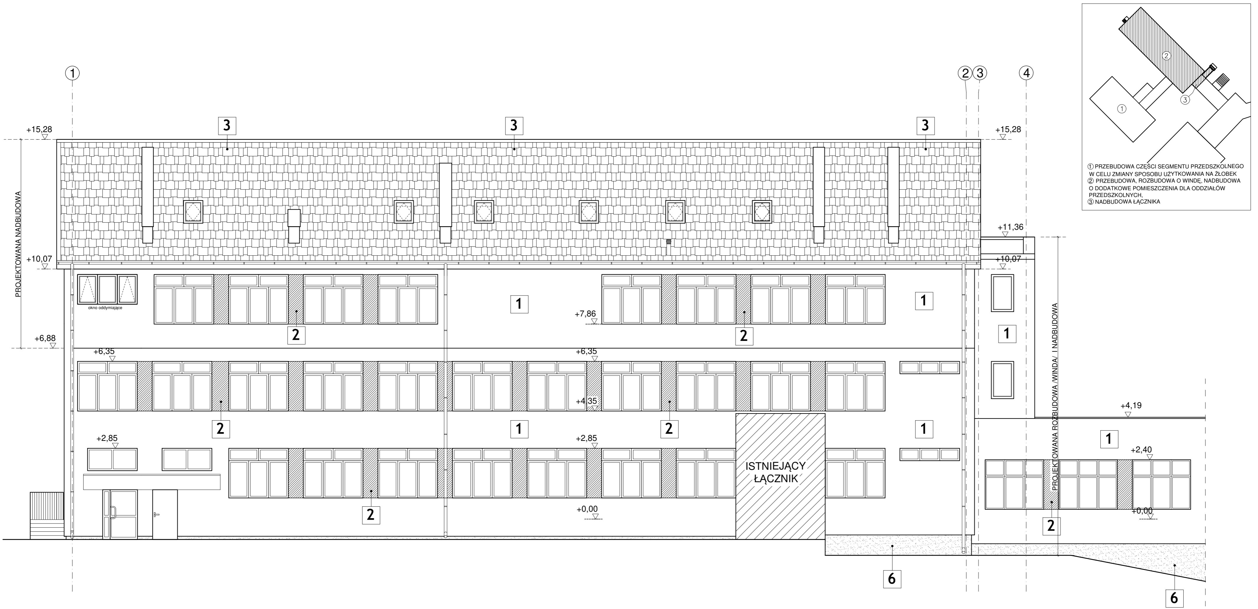
ELEWACJA POŁUDNIOWO - ZACHODNIA
